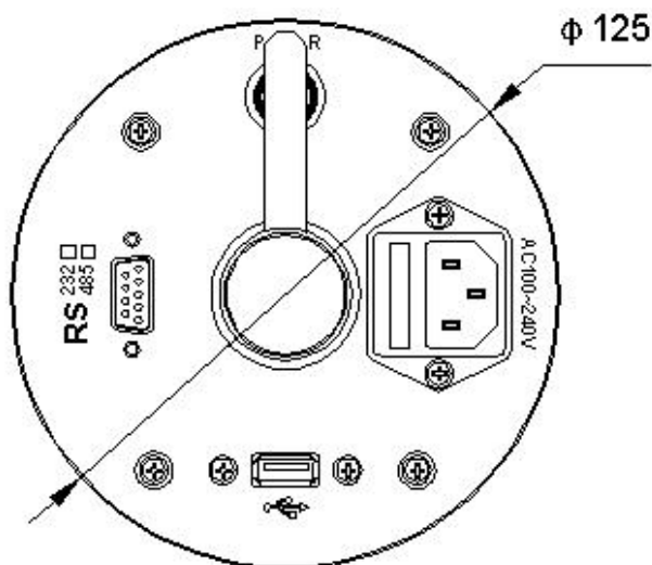
左视图
